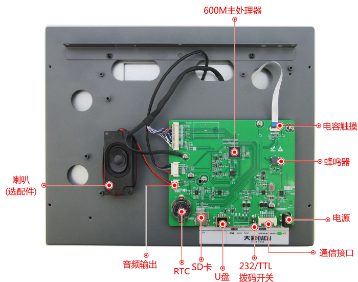
图 1-2 硬件配置图
