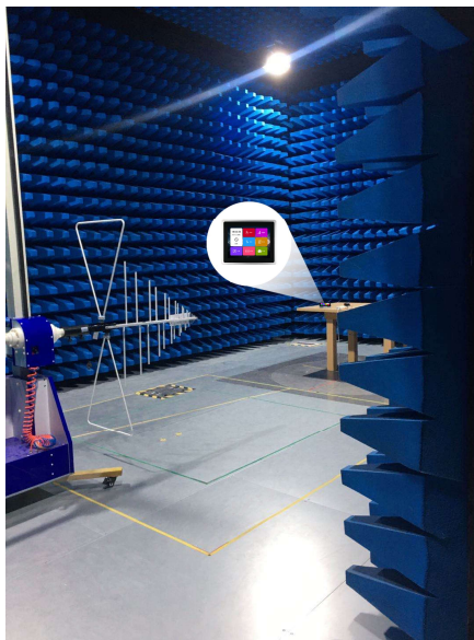
图 5-4 RE 测试图
