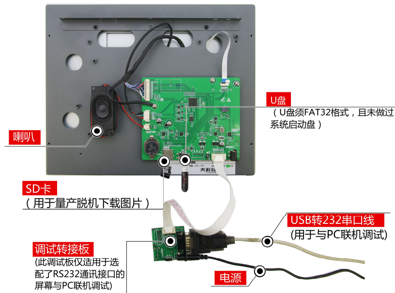
图 1-3 调试工具图
